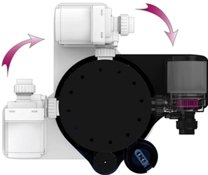
Fig. 2: A seconda dello spazio disponibile, la pompa può essere montata in diverse posizioni.
